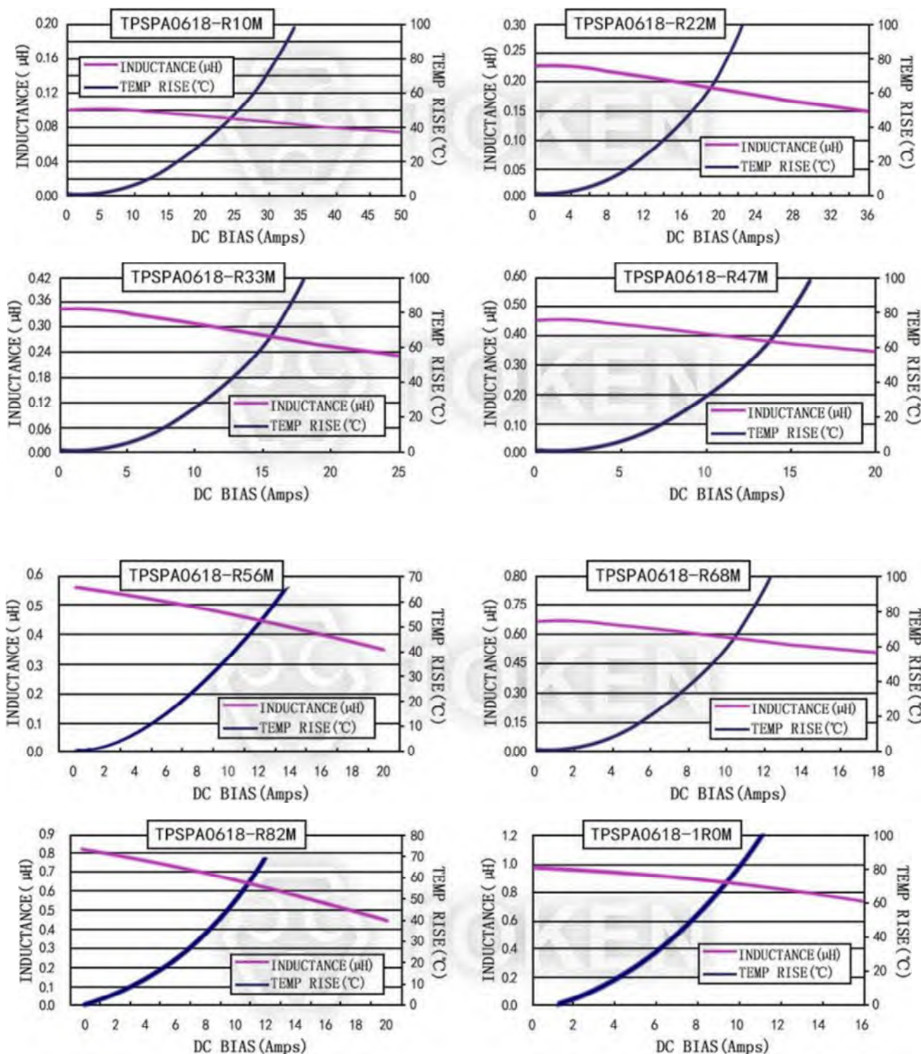
電流特性 TPSPA0618-***M 系列
