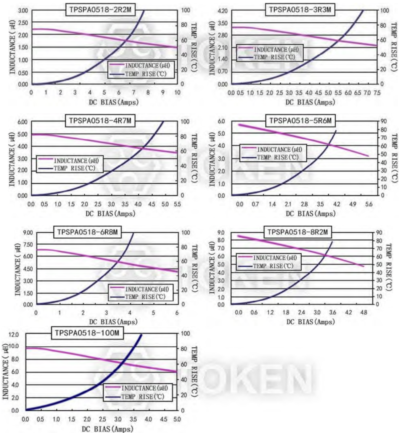
電流特性 TPSPA0518-***M 系列
