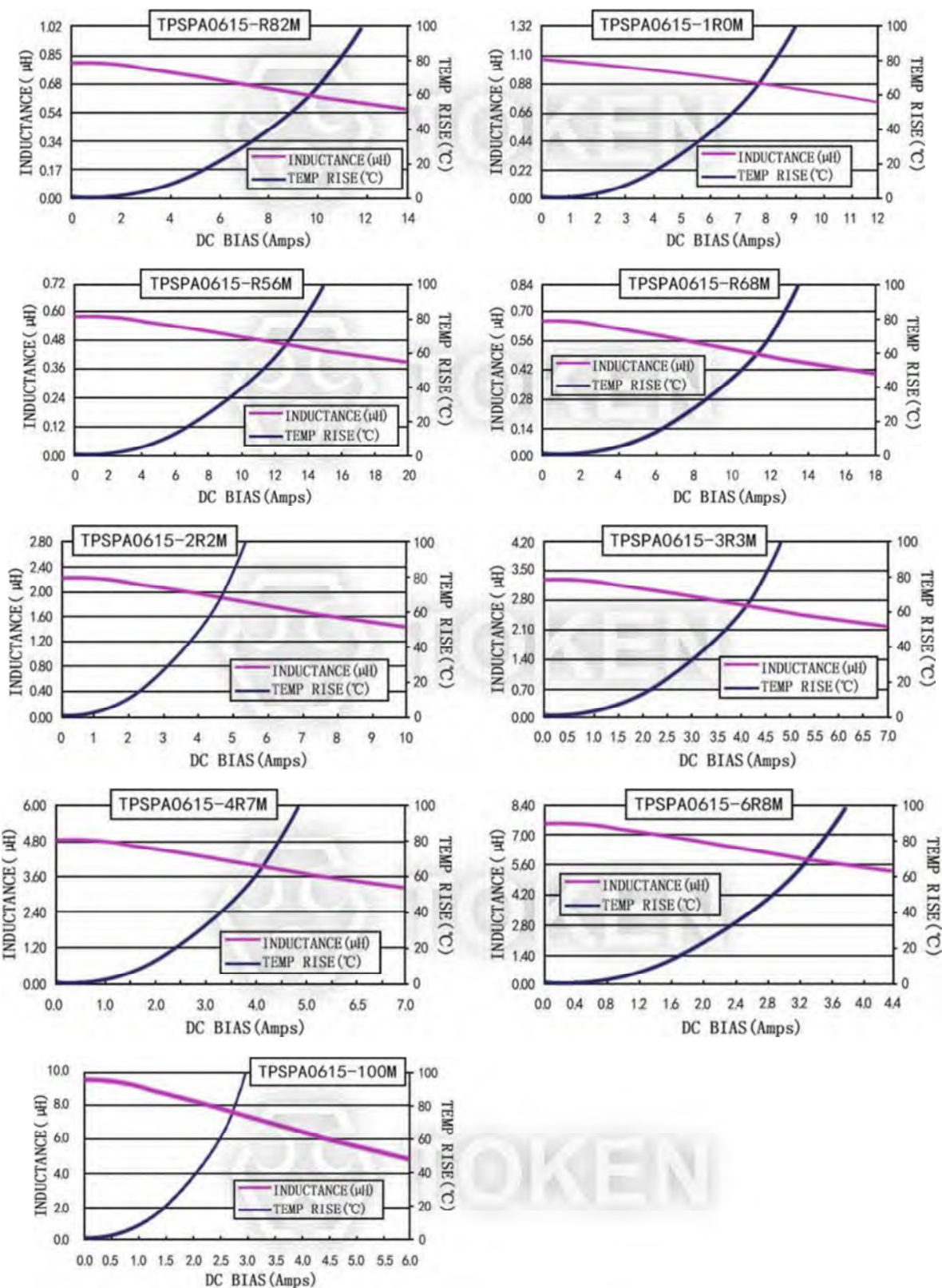
電流特性 TPSPA 0615-***M 系列
