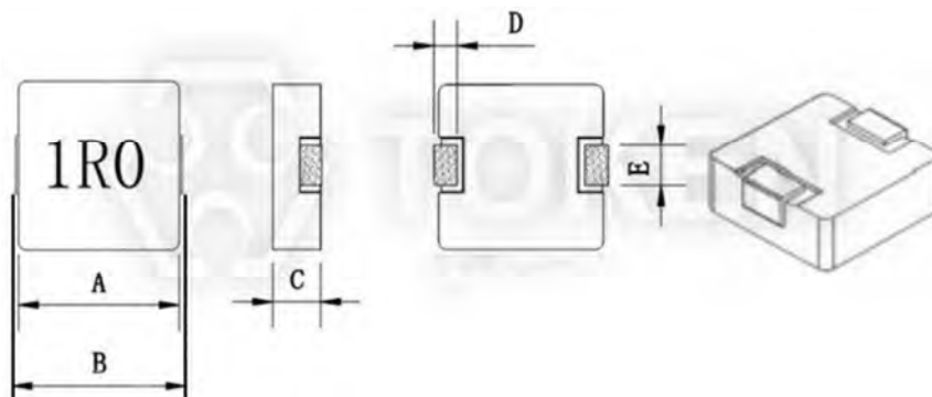
SMT 繞線大電流電感器 (TPSPA) 尺寸圖
