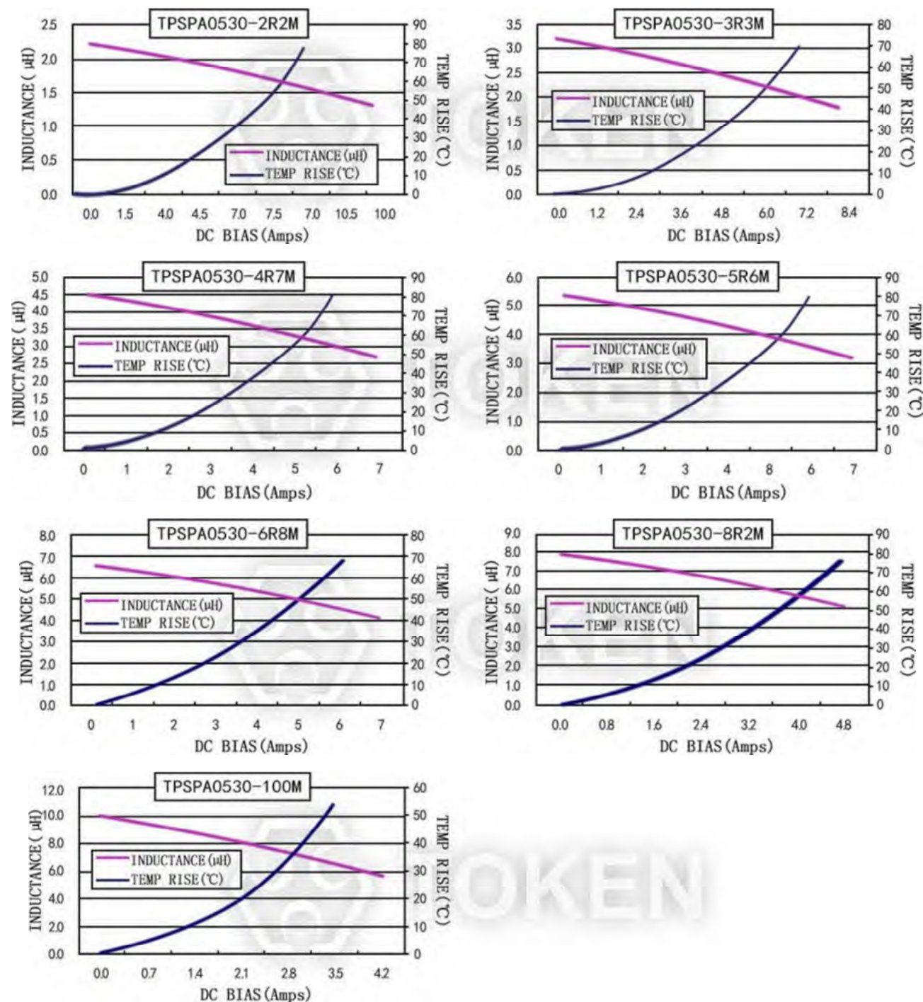
電流特性 TPSPA0530-***M 系列
