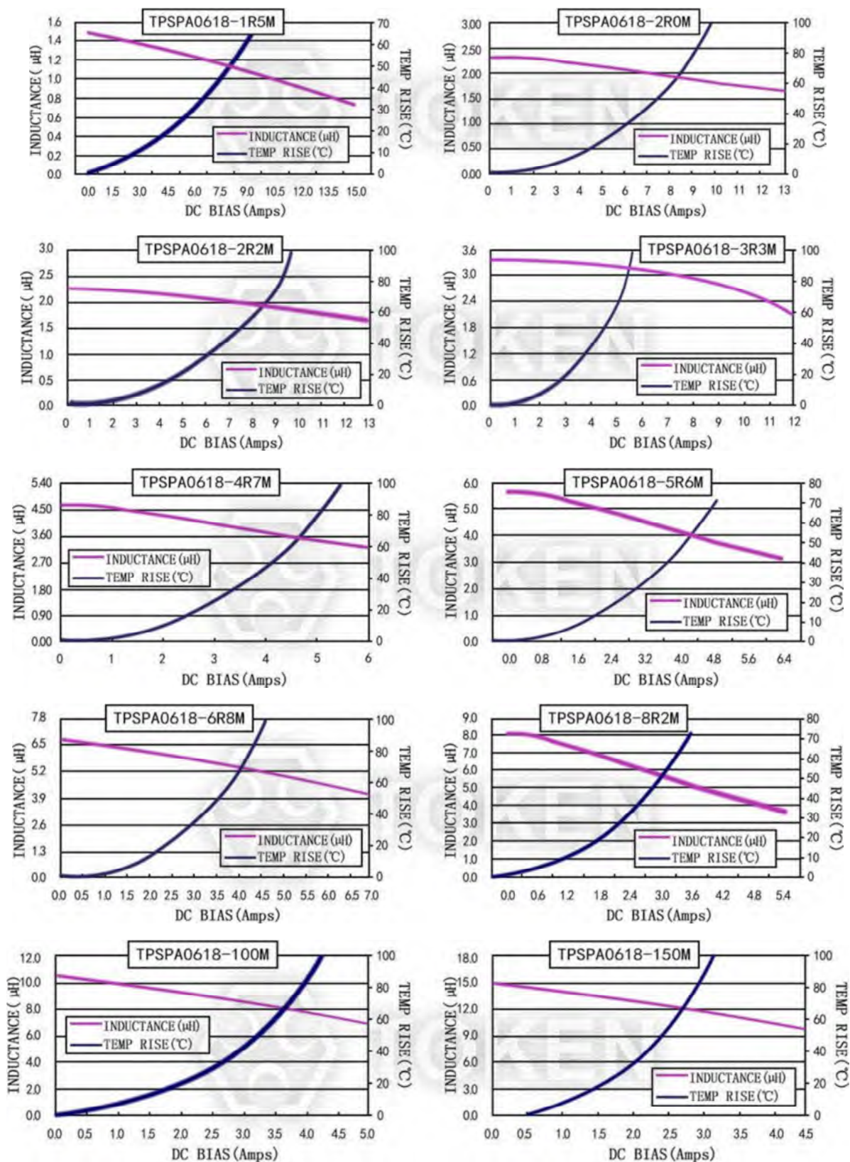
電流特性 TPSPA0618-***M 系列
