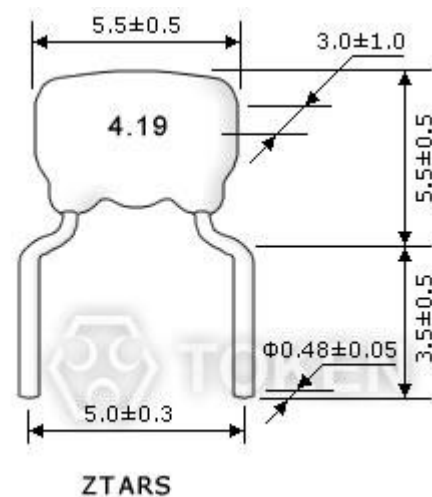
陶瓷諧振器 (ZTARS) 系列 尺寸圖
