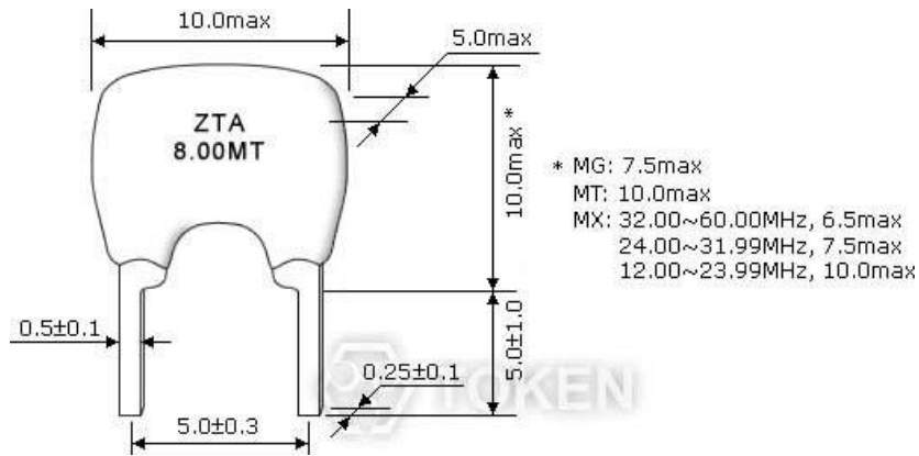
陶瓷諧振器 (ZTA8.00MT) 系列 尺寸圖
