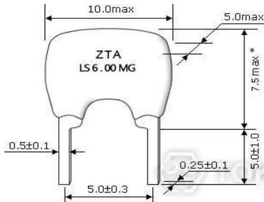
(ZTALS6.00MG) 系列 尺寸圖
