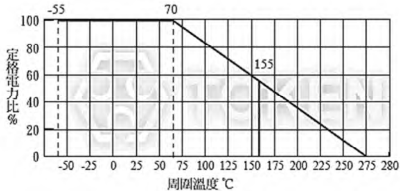
繞線無感電阻器 (KNPN) 降功率曲線
