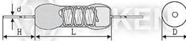
繞線無感電阻器 (KNPN) 尺寸規格圖
