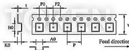
貼片電感線圈盤及編帶尺寸 (單位: mm)
