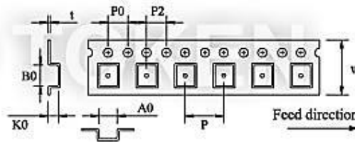
貼片電感線圈盤及編帶尺寸 (單位: mm)
