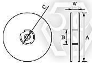
貼片電感線圈盤及編帶尺寸 (單位: mm)
