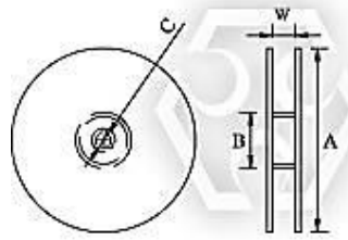
貼片電感線圈盤及編帶尺寸 (單位: mm)
