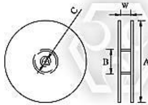
1. Reel Dimensions
