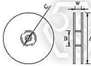
1. Reel Dimensions
