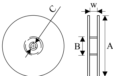
1. Reel Dimensions
