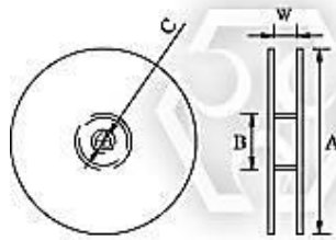
1. Reel Dimensions
